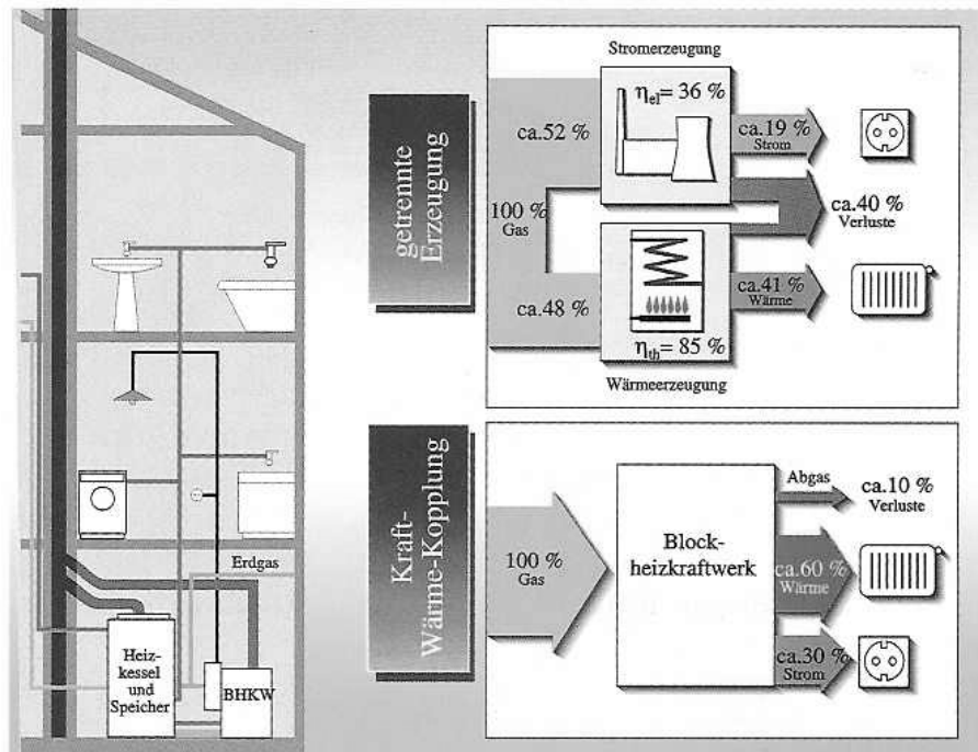
Die Grafik der ASUE vergleicht Energieverluste mit und ohne Kraft-Wärme-Kopplung.
